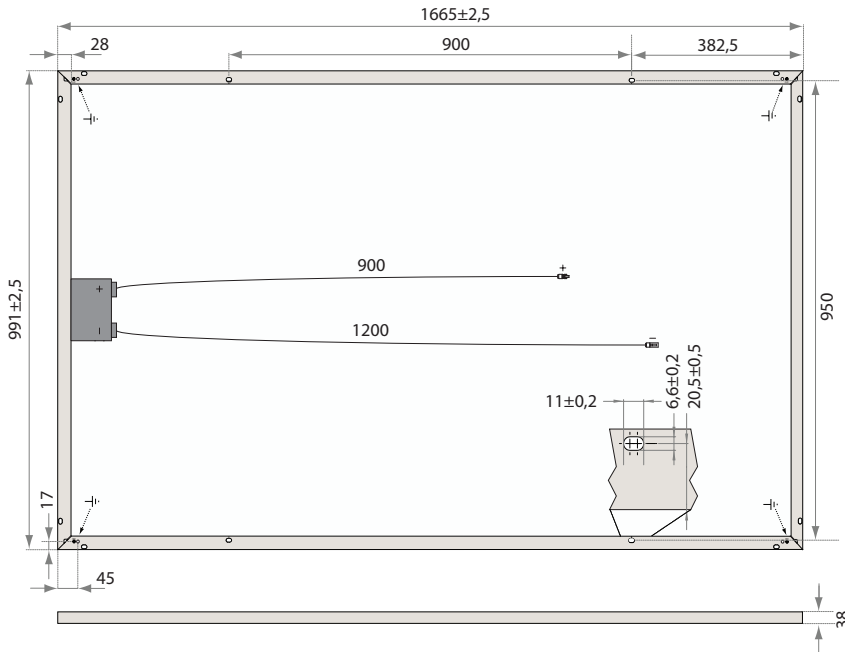
Abb. 24: Abmessungen: REC Peak Energy Serie
