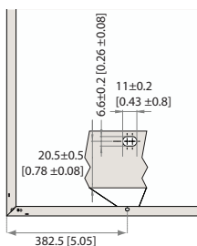
Abb. 7: Montagebohrungen: REC Peak Energy
