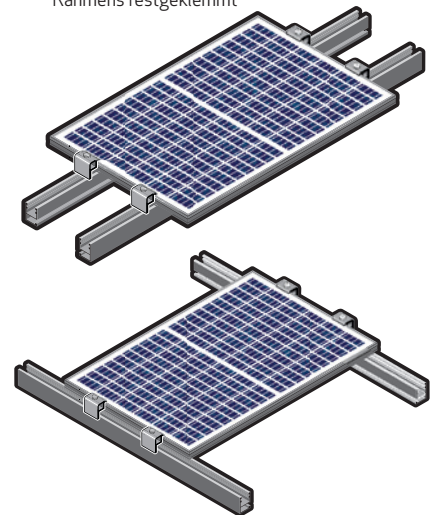
Abb. 3: Modulmontage: Schienen an der kurzen Seite des Rahmens festgeklemmt
