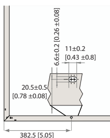
Abb. 11: Montagebohrungen: REC TwinPeak
