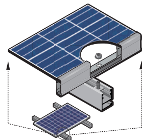
Abb. 9: Installation mithilfe der Montagebohrungen: REC Peak Energy
