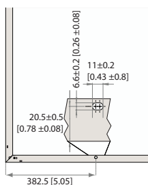
Abb. 15: Montagebohrungen: REC TwinPeak 2
