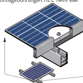
Abb. 13: Installation mithilfe der Montagebohrungen: REC TwinPeak
