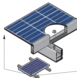
Abb. 17: Installation mithilfe der Montagebohrungen: REC TwinPeak 2
