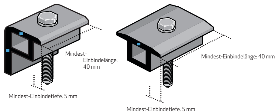
Abb. 4: Klemmenspezifikation: End- und Mittelklemmen
