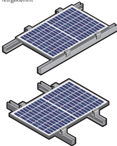
Abb. 2: Modulmontage: Schienen entlang des Rahmens festgeklemmt
