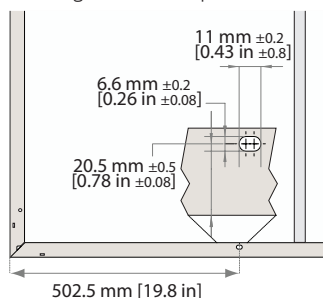
Abb. 12: Montagelöcher: REC Alpha 72 Serie
