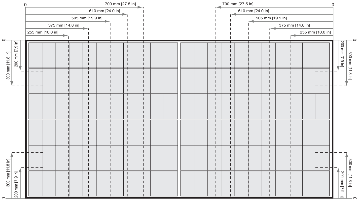
Abb. 6: Befestigen von REC Alpha Pure Serie Modulen auf Schienen parallel zur kurzen Seite des Moduls
