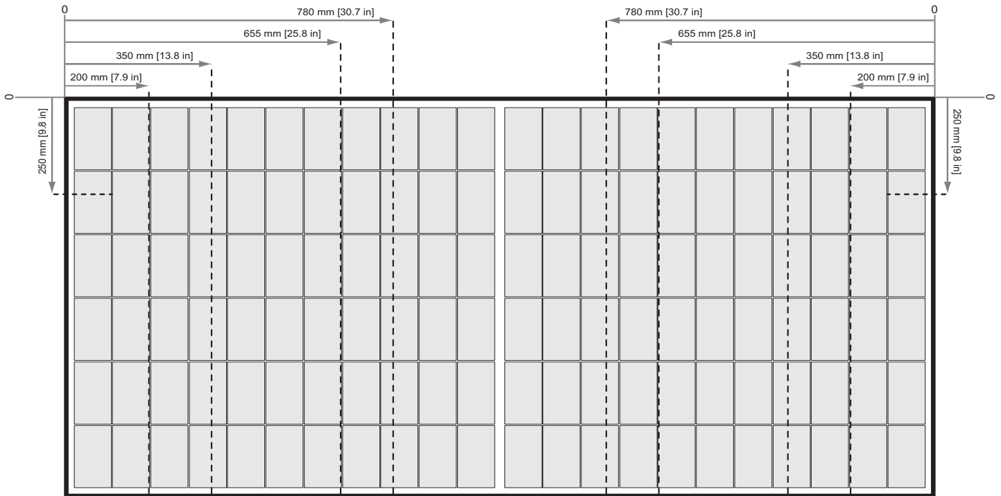
Abb. 9: Befestigen von REC Alpha 72 Serie Modulen auf durchlaufenden Schienen parallel zur kurzen Seite des Moduls
