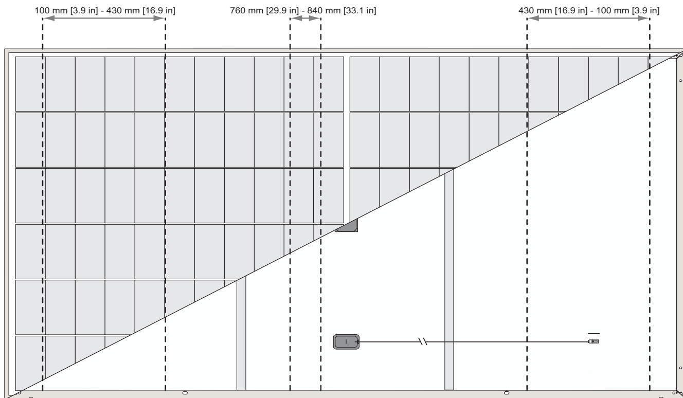
Abb. 24: Sechs-Punkt-Montage Klemmzonen
