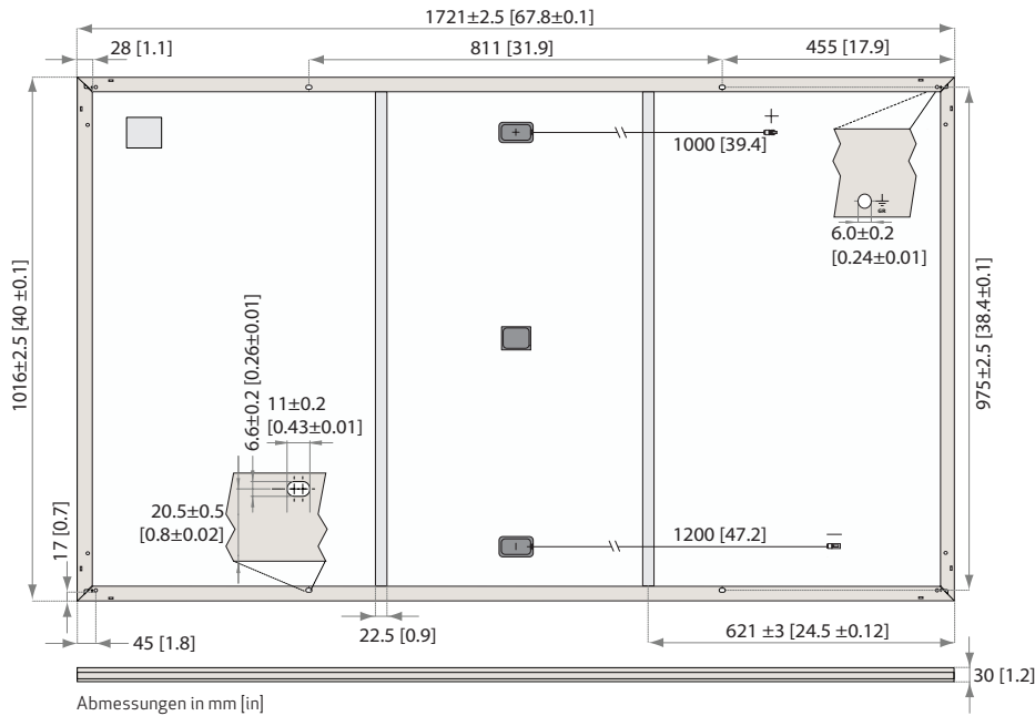
Abb. 18: Abmessungen: REC Alpha Serie
