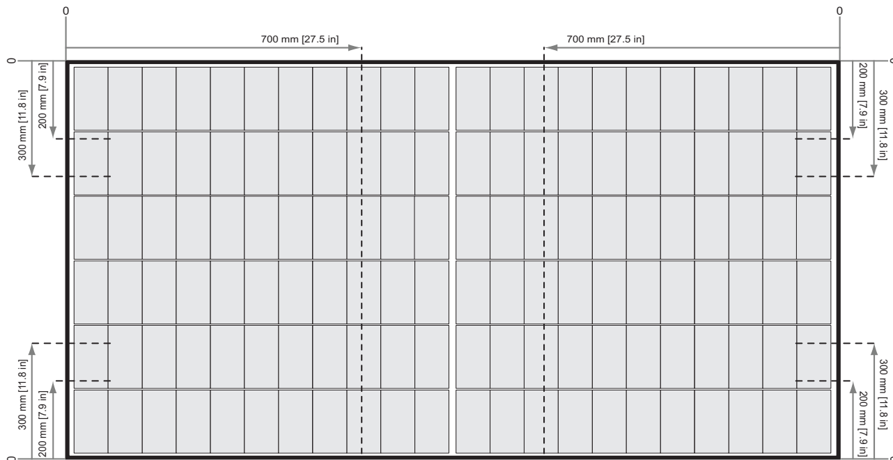
Abb. 7: Befestigen von REC Alpha Pure Serie Modulen auf Schienen parallel zur langen Seite des Moduls
