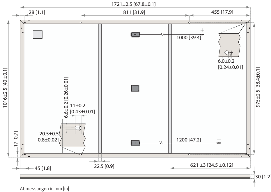
Abb. 19: Abmessungen: REC Alpha Black Serie
