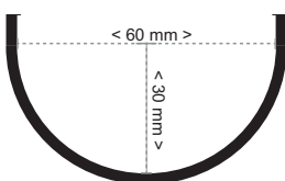
Abb. 16: Mindest-Biegeradius der Kabel
