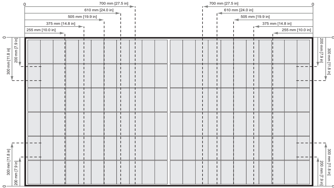
Abb. 8: Befestigen von REC Alpha Pure Serie Modulen mit Kurzschienen
