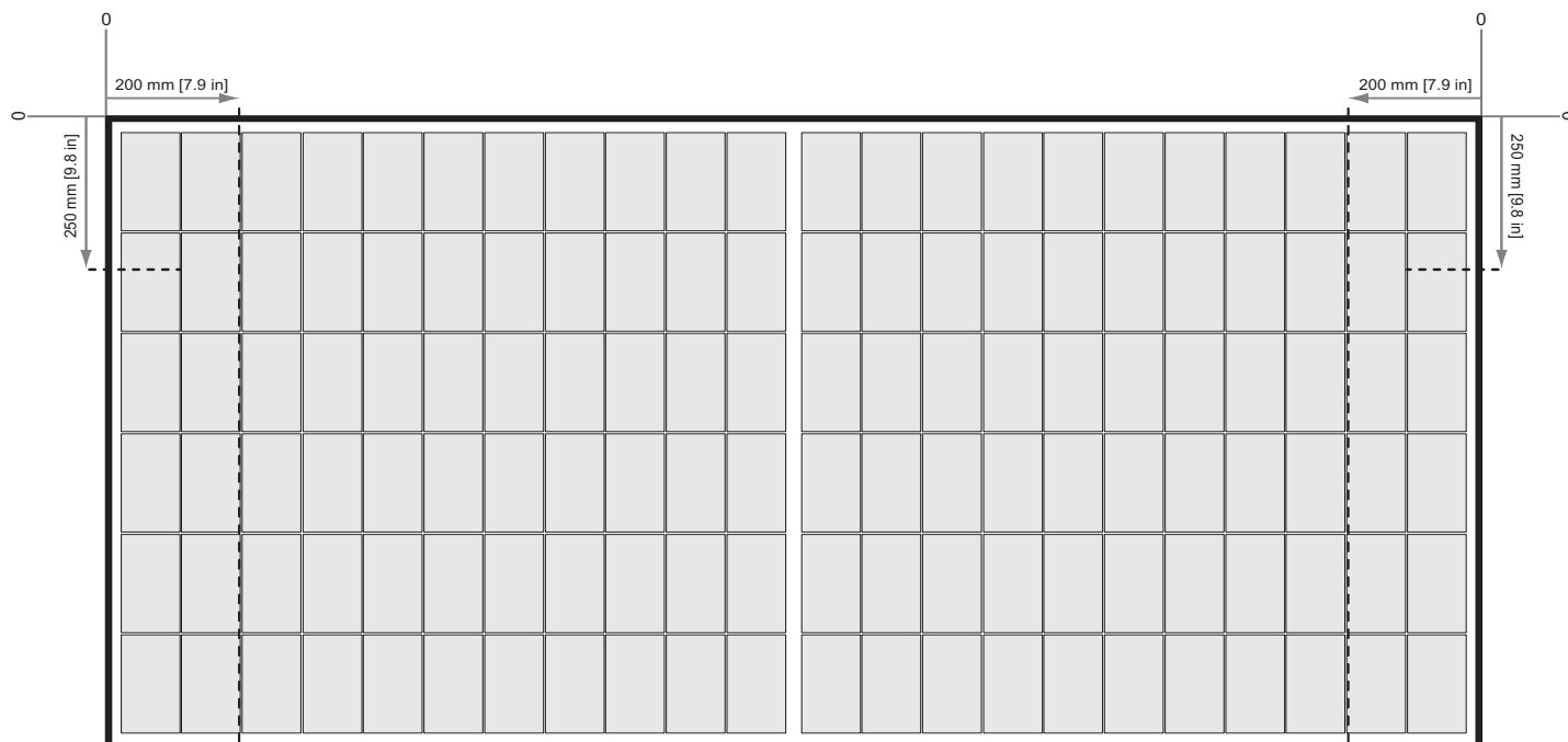
Abb. 10: Befestigen von REC Alpha 72 Serie Modulen auf Kurzschienen parallel zur kurzen Seite des Moduls
