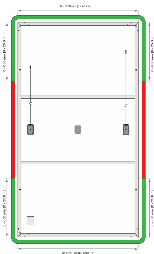
Abb. 23: MLPE-Geräte Installationsbereiche: REC Alpha 72 Serie
