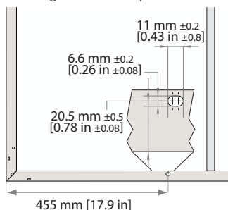
Abb. 11: Montagelöcher: REC Alpha Serie
