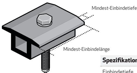
Abb. 1: Klemmenspezifikation
